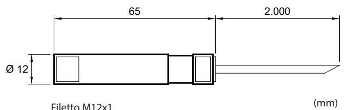
Filetto M12x1
