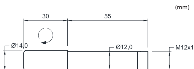
Filetto M12x1
