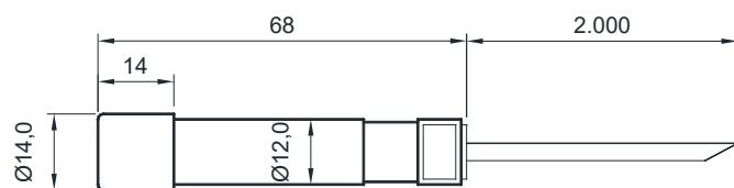
Dimensioni art. SM313002 (***) (mm)
